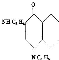
Rosindulin.
